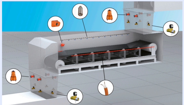
Protection Convoyeur
